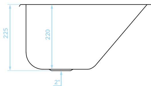
PRZEKRÓJ A-A
